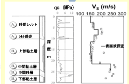
ボーリング情報との比較
