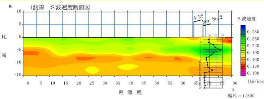
S波速度構造断面図
