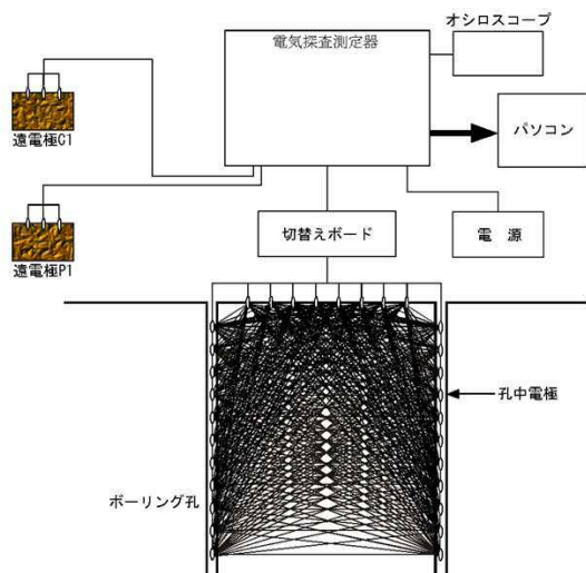
比抵抗トモグラフィーの測定概念図
